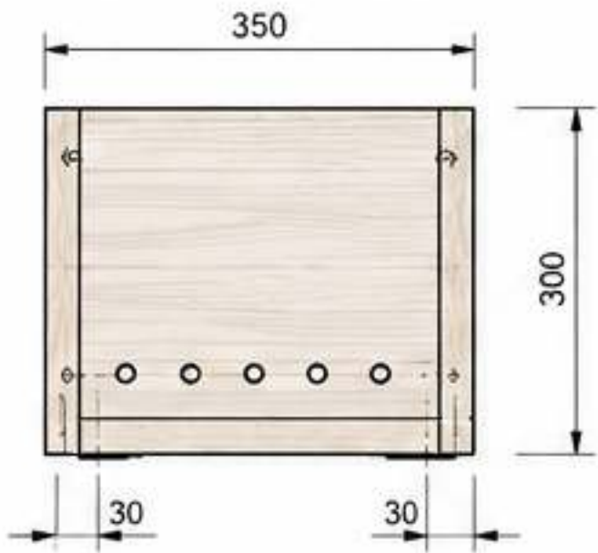
ZIJAAANZICHT (korte zijde)
