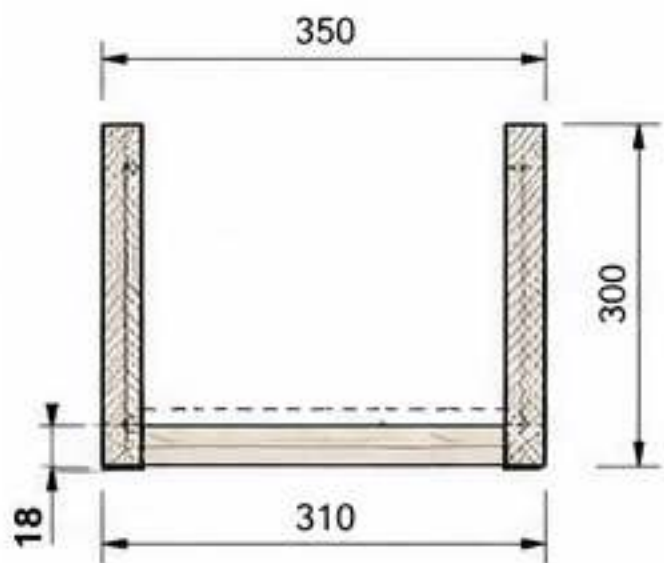
DOORSNEDE A-A (dwars)
