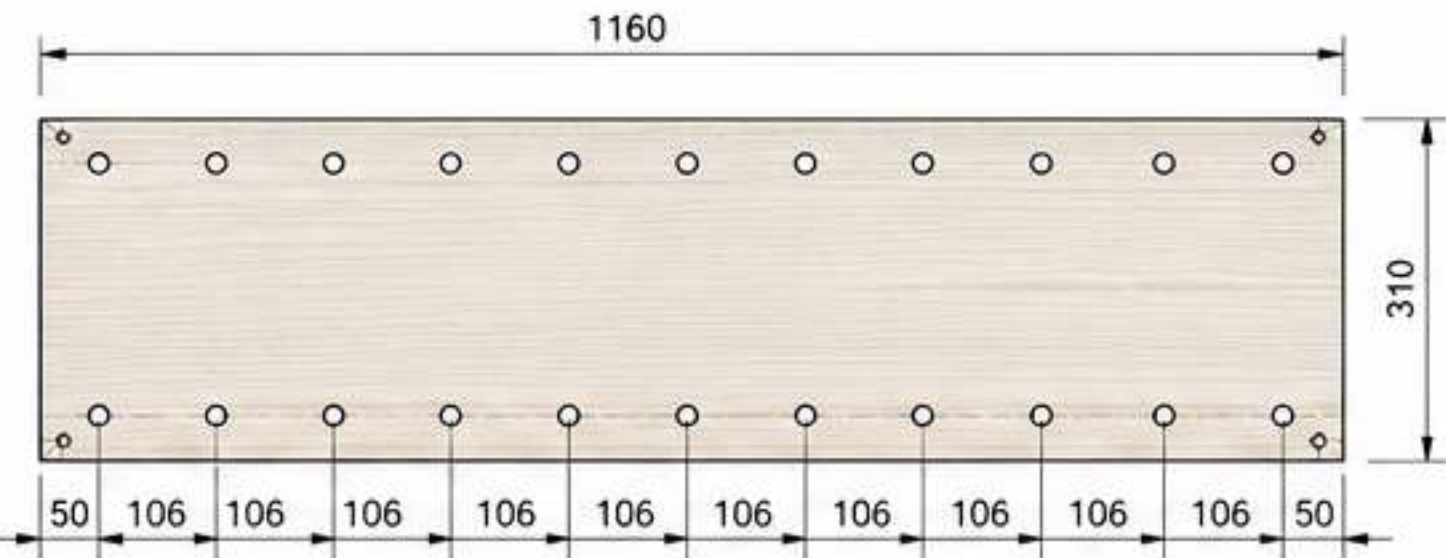
ONDERAANZICHT (bodemplaat)
