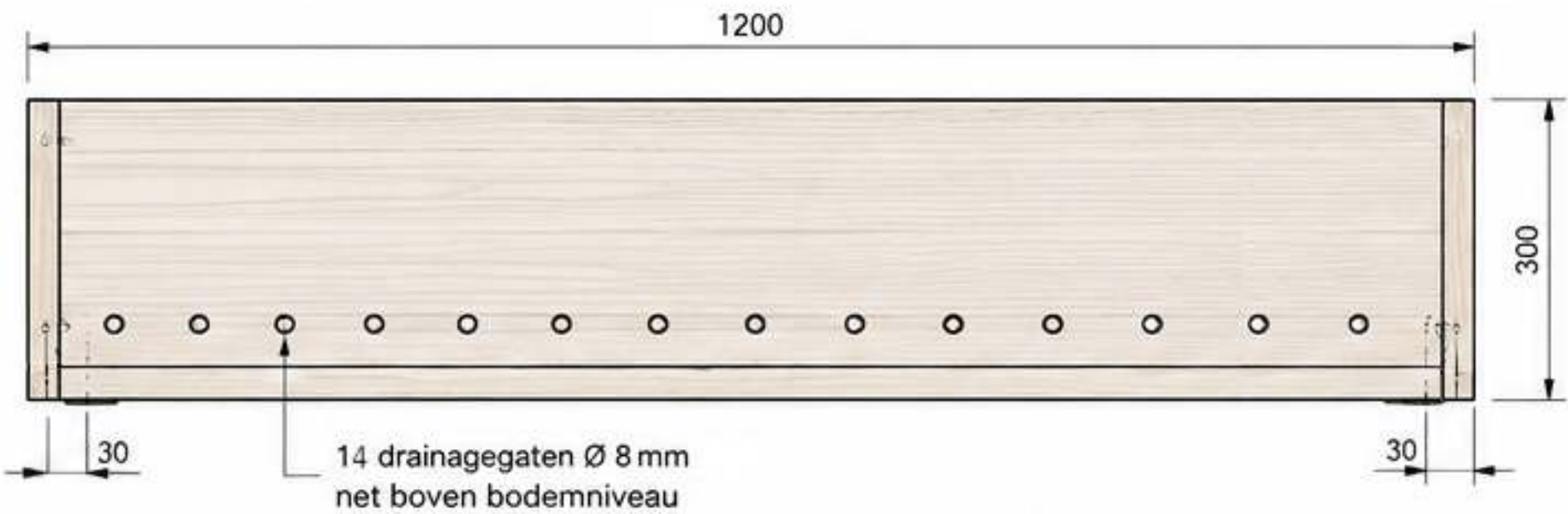
VOORAANZICHT (lange zijde)
