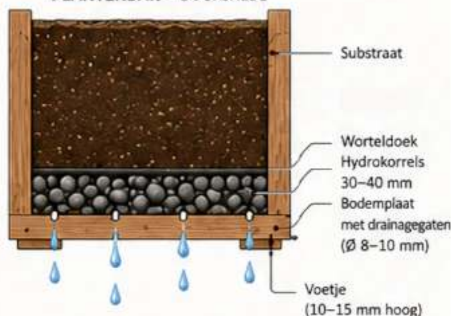
PLANTENBAK – DOORSNEDE
