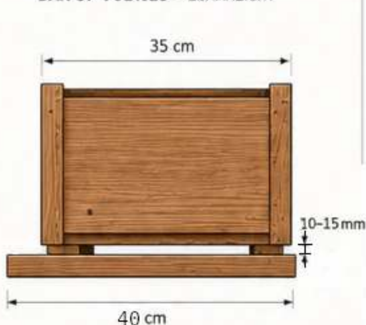
BAK OP VOETJES – ZIJAAANZICHT
