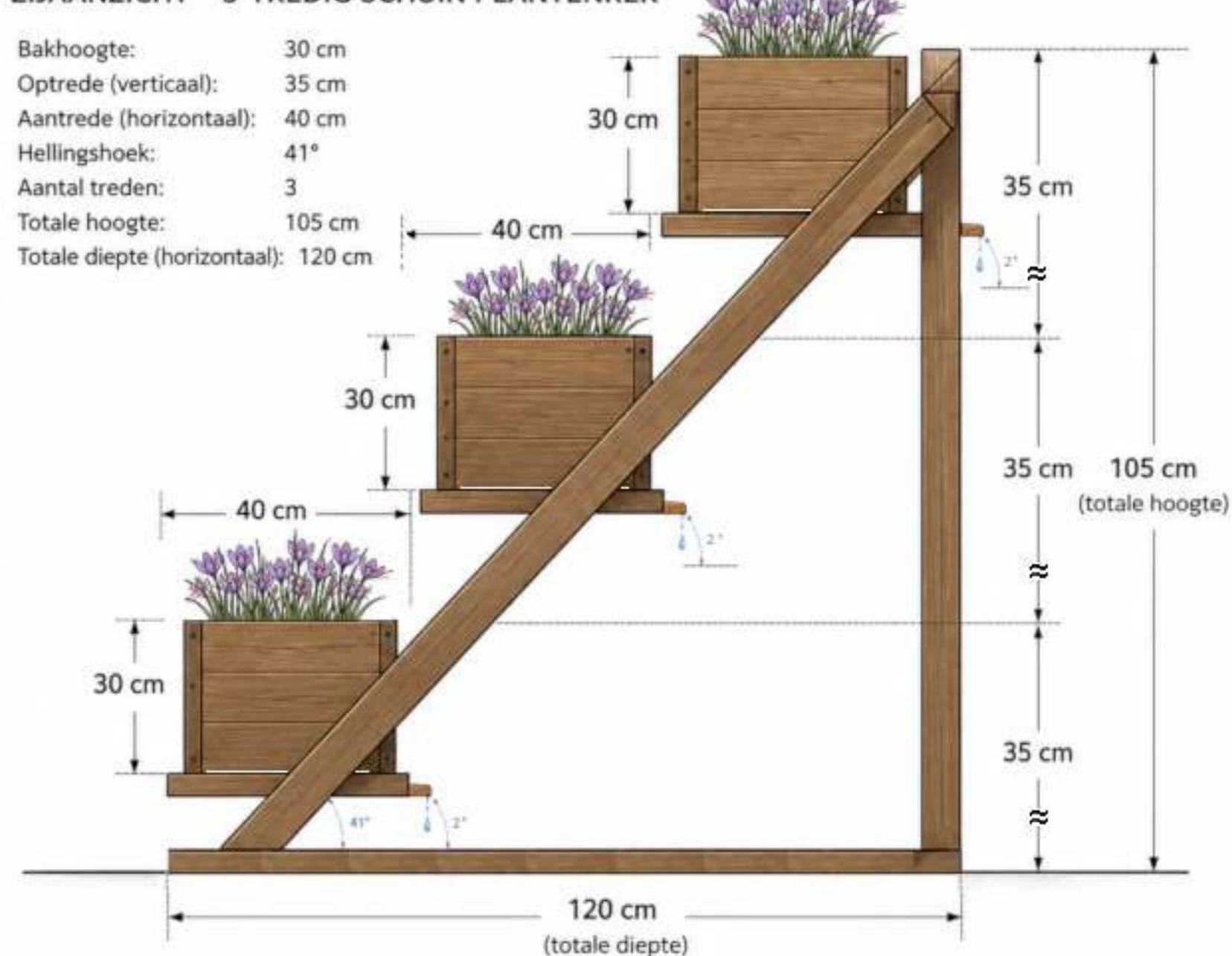
ZIJAAANZICHT – 3-TREDIG SCHUIN PLANTENREK
